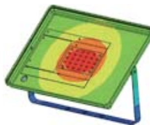
Distribución Térmica
